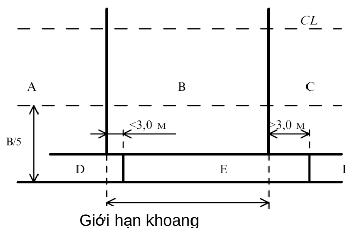
Hình 9/4.3.5-1 Giải định ngập
