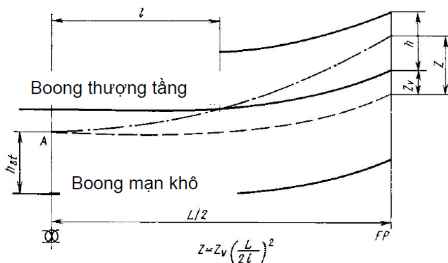
Hình 11/4.3.1-8(1) Thương tầng chạy suốt chiều dài có chiều cao lớn hơn tiêu chuẩn
