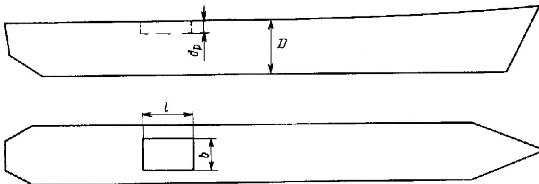
Hình 11/4.4.9-1 Hiệu chỉnh hõm ở boong mạn khô
