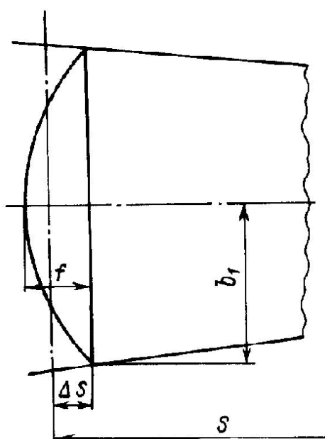
Hình 11/4.2.2-2 Vách mút thượng tầng nhô
