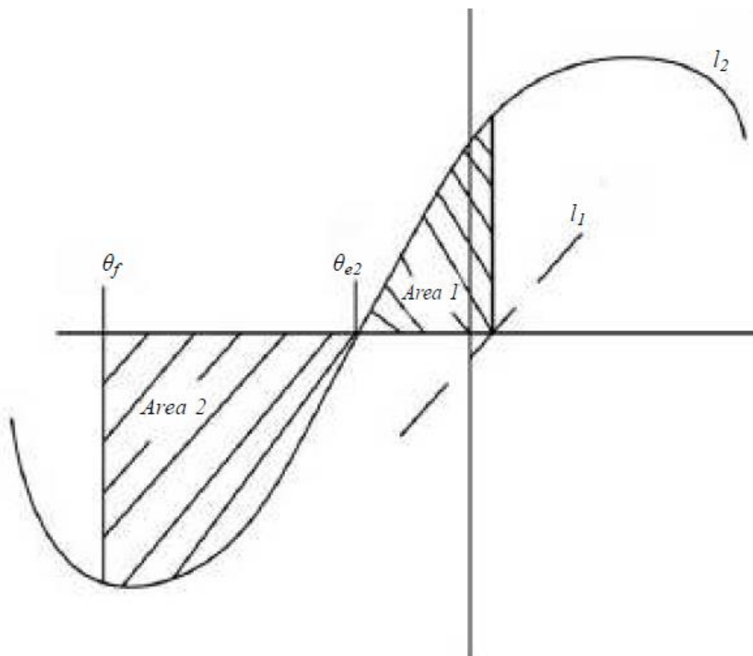
Hình 10/4.1.5-1 Ổn định khi hàng rơi
